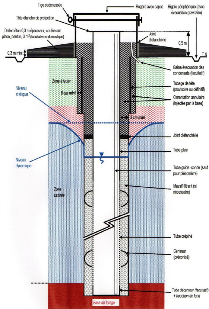
Figure 16 — Exemple de protection de la tête de forage (Source documentaire : BRGM)
